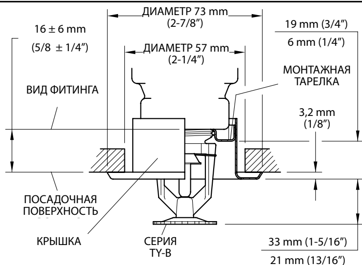
РИС. 6 ЗАГЛУБЛЕННЫЙ СПРИНКЛЕР С ПЛОСКОЙ РОЗЕТКОЙ СЕРИИ TY-B В СБОРЕ С ДВУХСЕКЦИОННЫМ ЗАГЛУБЛЕННЫМ ПОДРОЗЕТНИКОМ ОБЩЕЙ НАСТРОЙКИ 19 mm (3/4"), ТИПА 40, K=115, 3/4" NPT
