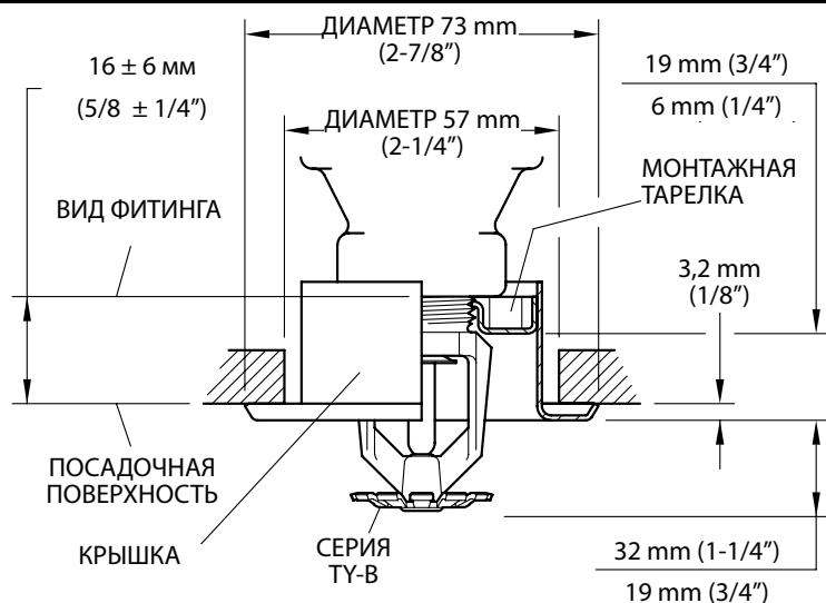
РИС. 5 ЗАГЛУБЛЕННЫЙ СПРИНКЛЕР С ПЛОСКОЙ РОЗЕТКОЙ СЕРИИ TY-B В СБОРЕ С ДВУХСЕКЦИОННЫМ ЗАГЛУБЛЕННЫМ ПОДРОЗЕТНИКОМ ОБЩЕЙ НАСТРОЙКИ 19 mm (3/4"), ТИПА 10, K=80, 1/2" NPT
